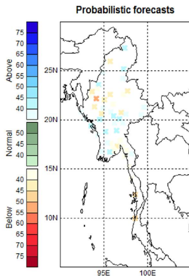
ECHAM_gph_Apr_JJAS
