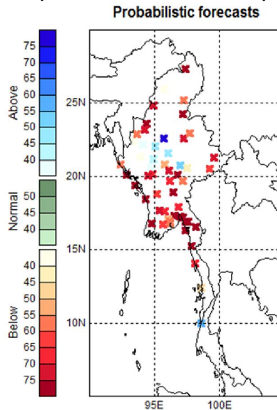
ECHAM_gph_Apr_JJAS
