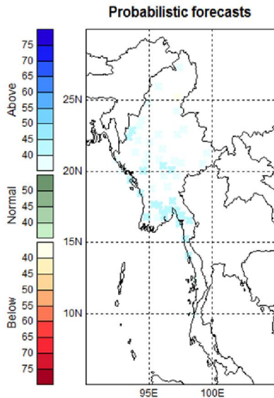
ECHAM_pptn_Apr_JJAS
