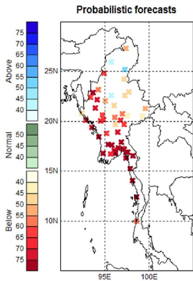
ECHAM_pptn_Apr_JJAS
